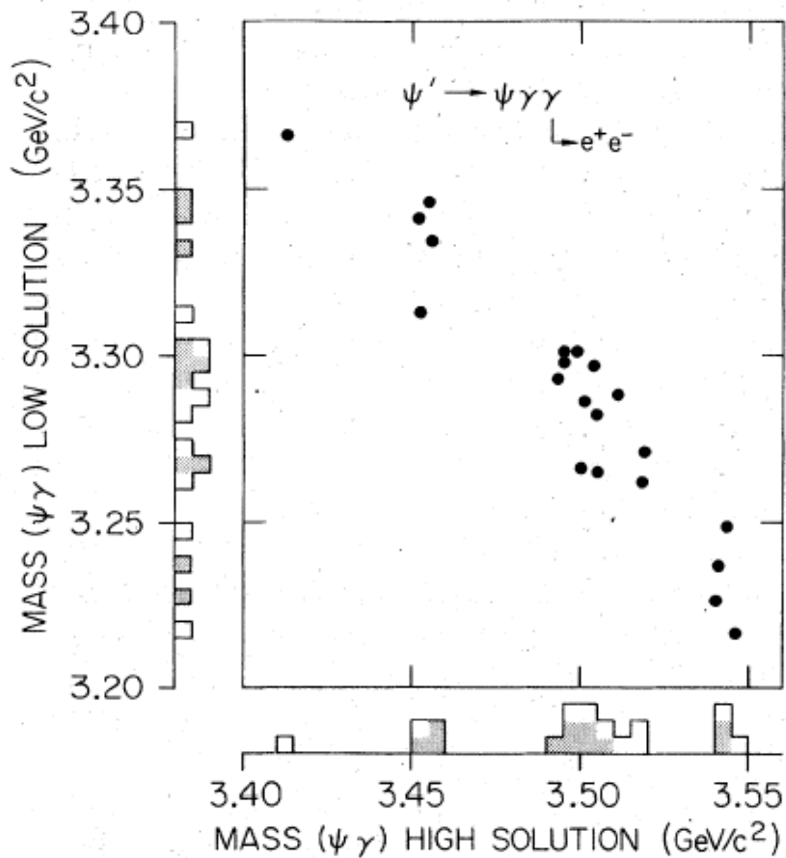
SLAC-LBL Mark I experiment
